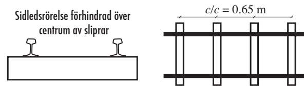
figur 2 Tvärsnitt och vy ovanifrån av en del av en spårsektion.
