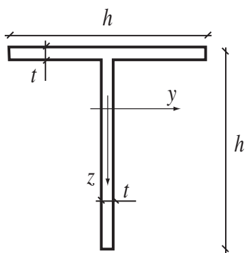
figur 2 Tunnväggigt T-tvärsnitt utsatt för böjande moment, M_y och tvärkraft T_z .
